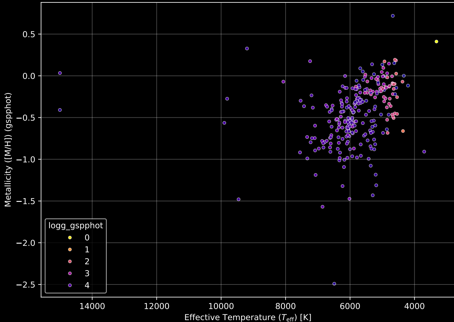
GALAH DR4 Field: [3545] Stellar Population Parameters (n= 263)
