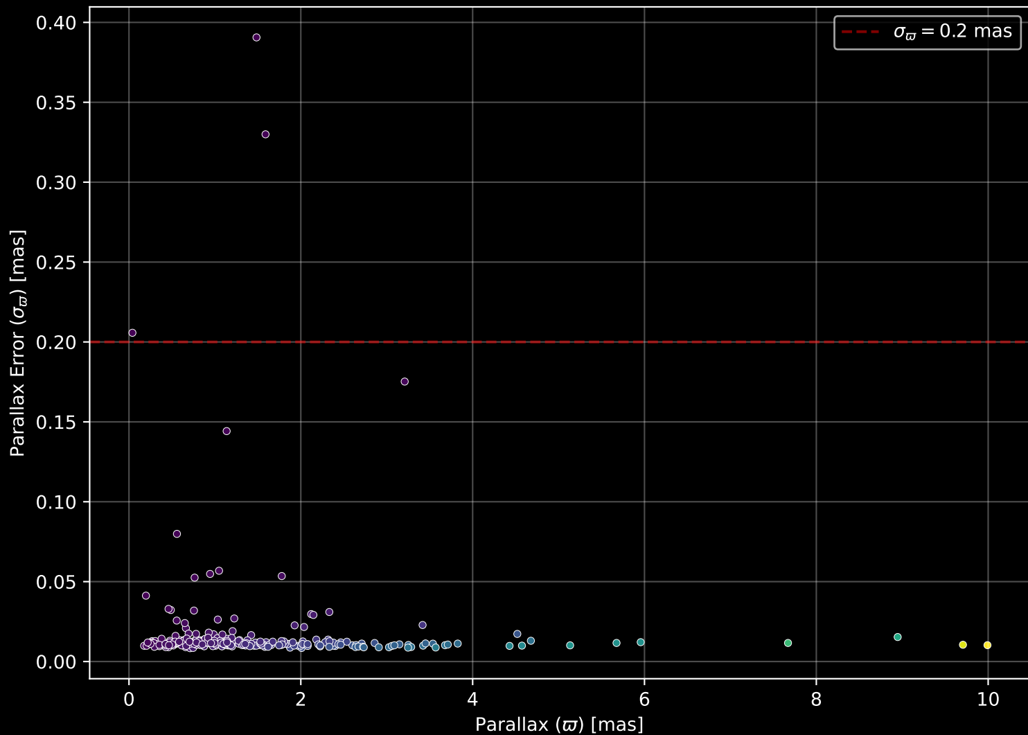
GALAH DR4 Field: [3545] Parallax Quality (n= 263)
