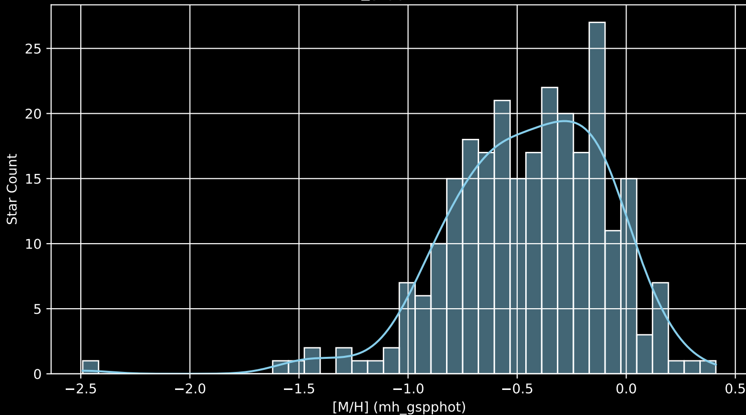
GALAH DR4 Field: [3545] [M/H] (mh_gspphot) (n= 262)
